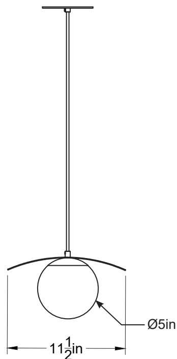
Côté/Side
