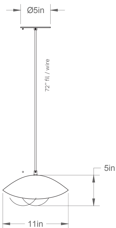
Avant/Front
