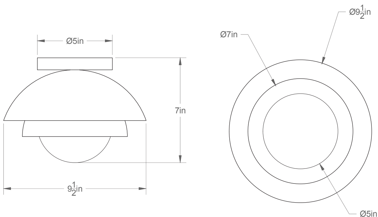
Avant/Front
