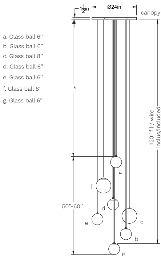
Avant/Front
