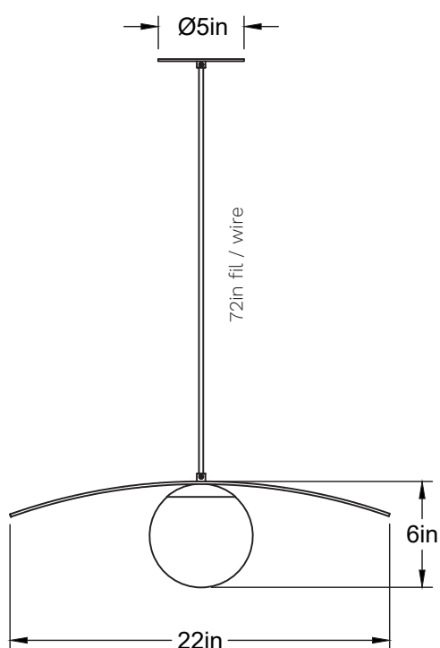
Avant/Front
