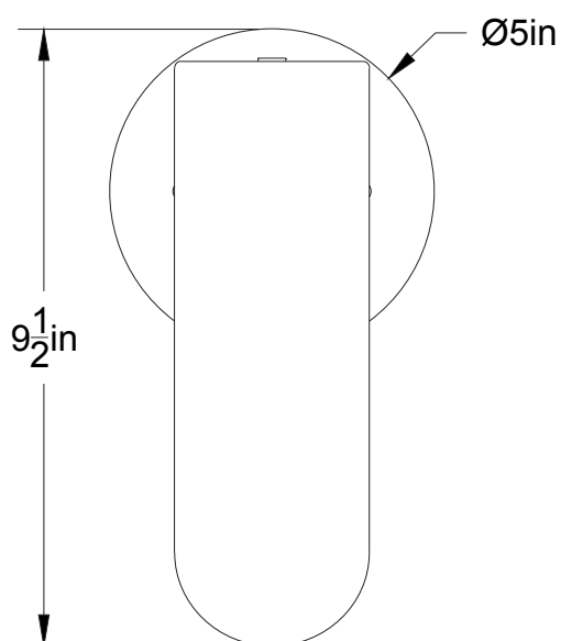
Avant/Front
